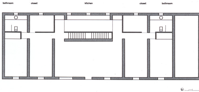
34 · PLANTA BAJA
